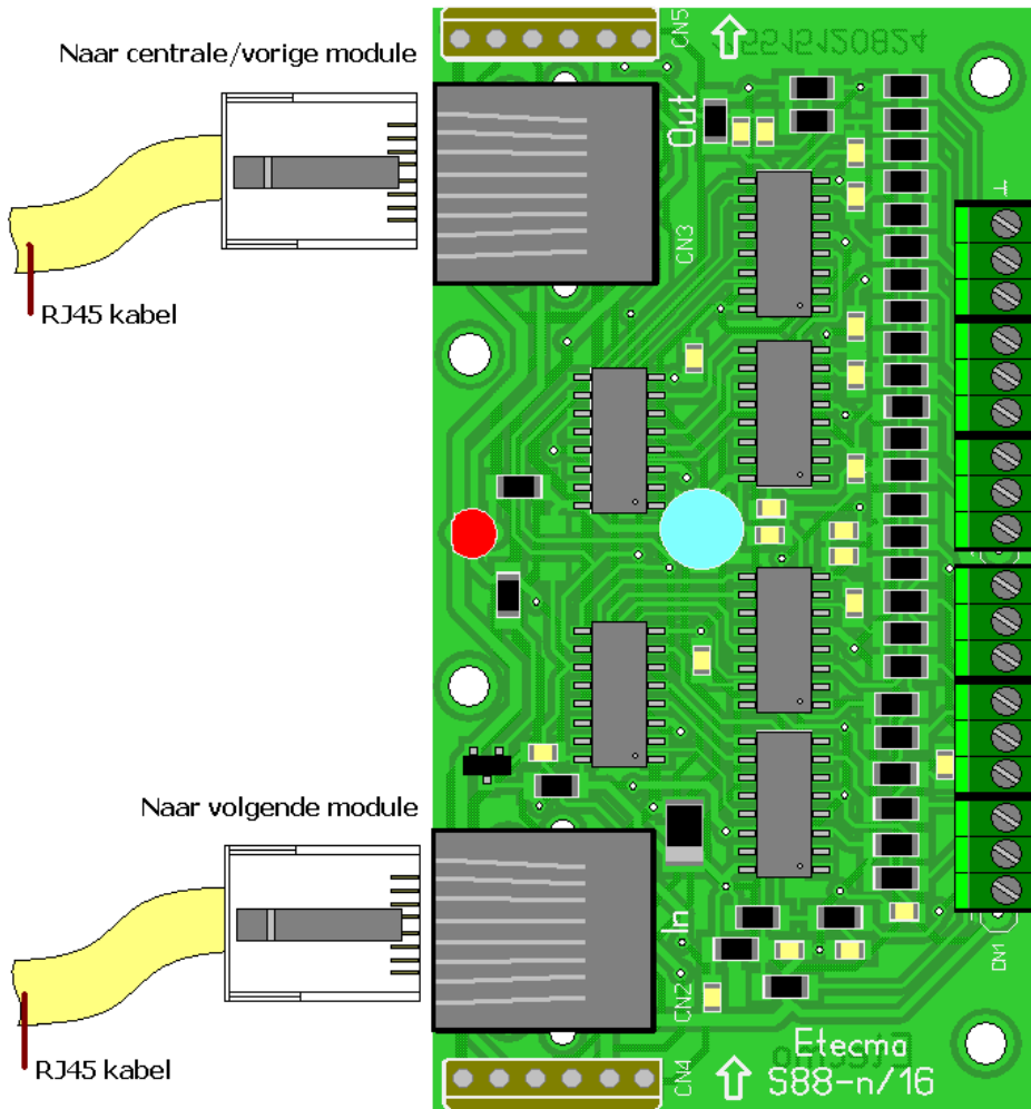
Aansluiting volgens s88-N standaard
