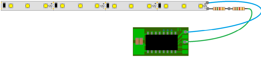
Aansluiten van een LED strip aan de decoder met extra voorschakelweerstand.
