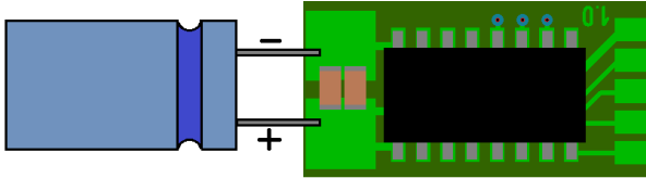
Aansluiten van extra buffer condensator (<math><100\mu F</math>).
