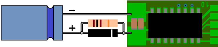
Aansluiten van extra buffer condensator (>math>>100\mu F</math>), Weerstand = 100 ohm, diode is 1N4001.
